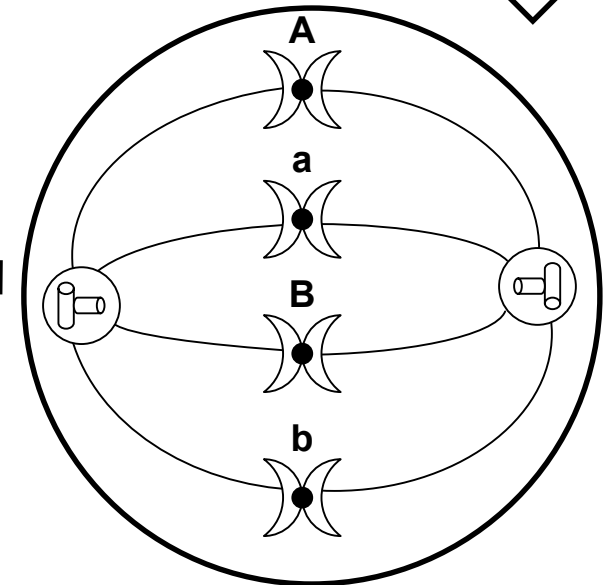
Metaphase
