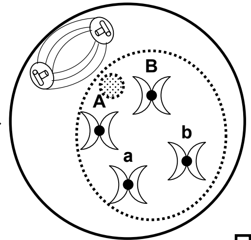
Metaphase
